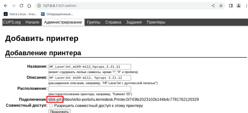
Рисунок 20 – Проверка URL
