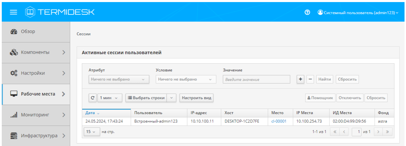
Рисунок 57 – Просмотр сведений об активных сессиях пользователей в фондах ВРМ
