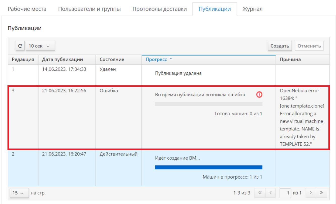
Рисунок 54 – Индикация возникновения ошибки при публикации
