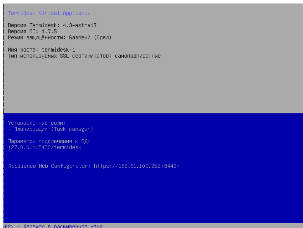
Рисунок 20 – Окно управления ВМТ
