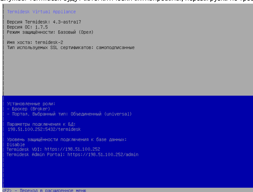
Рисунок 43 – Окно управления ВМТ
