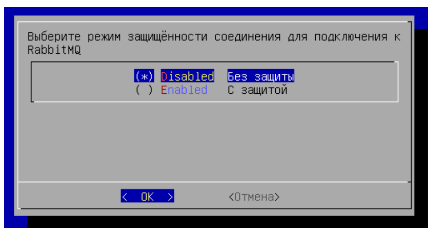
Рисунок 93 – Выбор протокола для подключения к RabbitMQ
