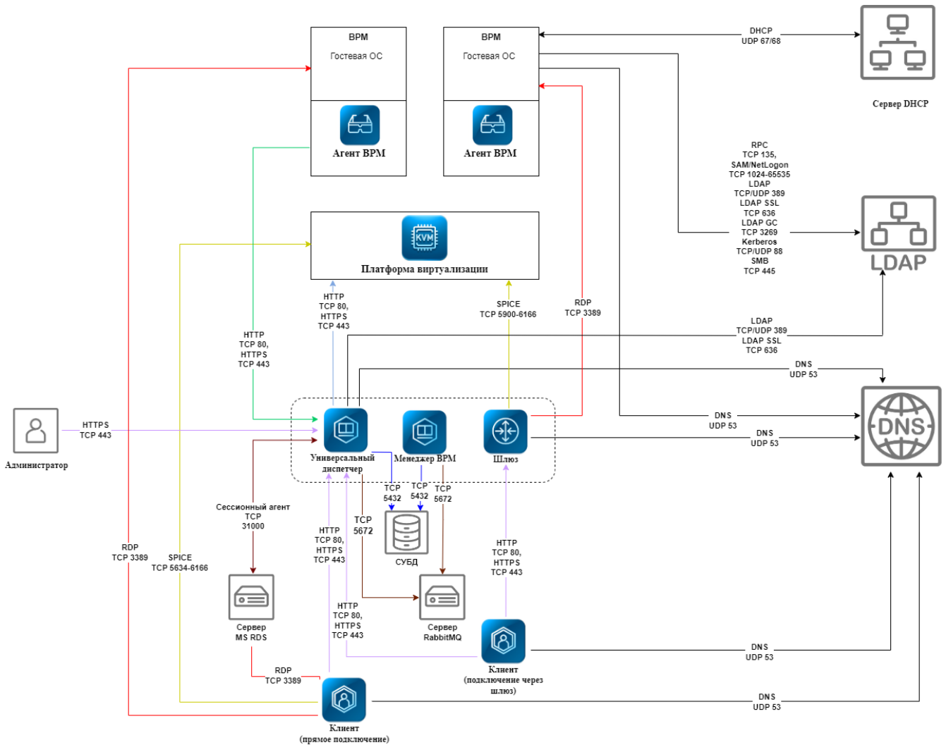
Рисунок 2 – Схема сетевого взаимодействия компонентов Termidesk
