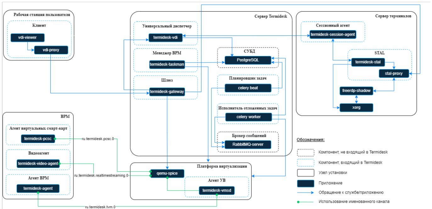
Рисунок 1 – Схема взаимодействия компонентов и процессов
