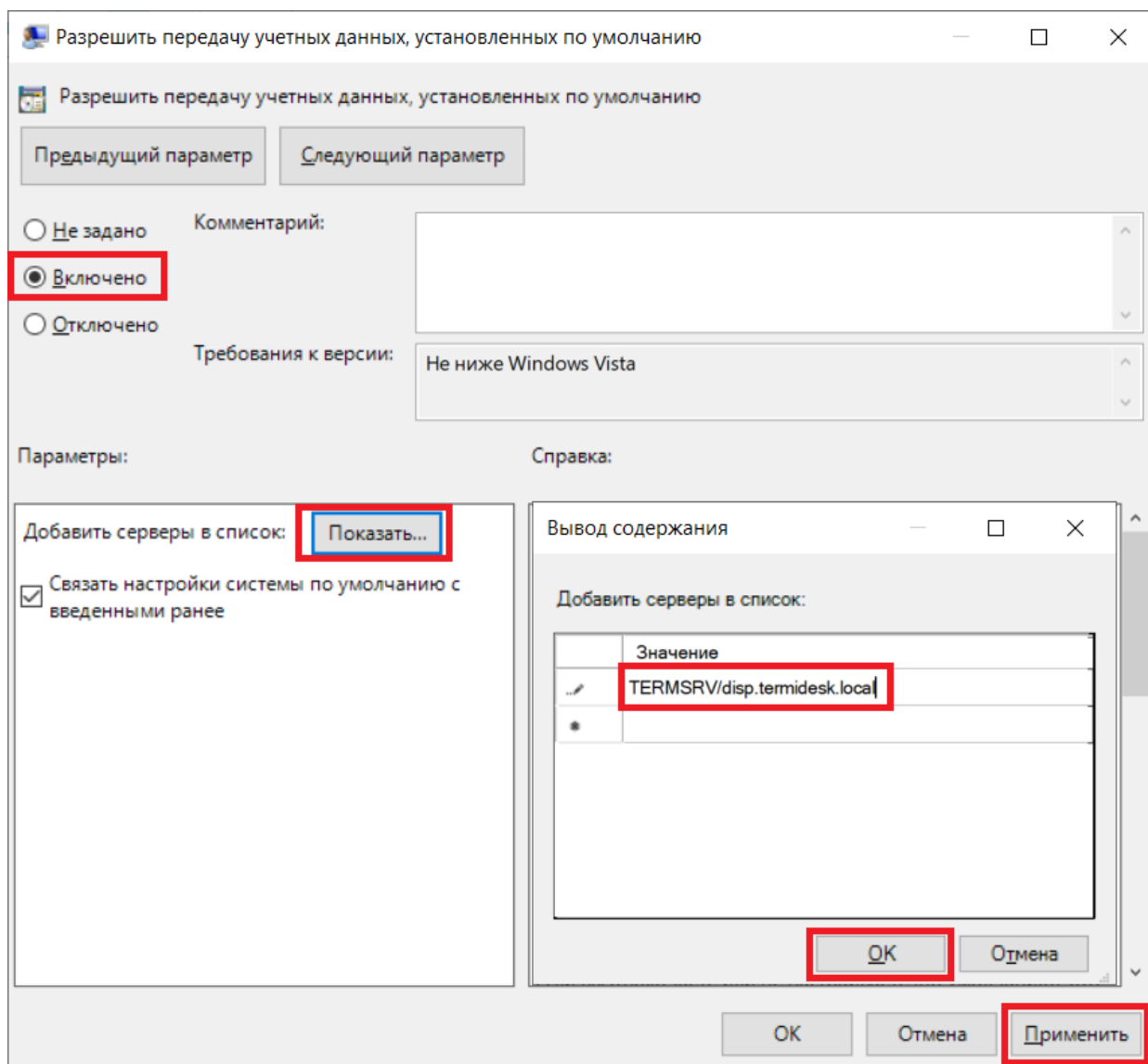
Рисунок 15 – Редактирование параметра «Разрешить передачу учетных данных, установленных по умолчанию» групповых политик
