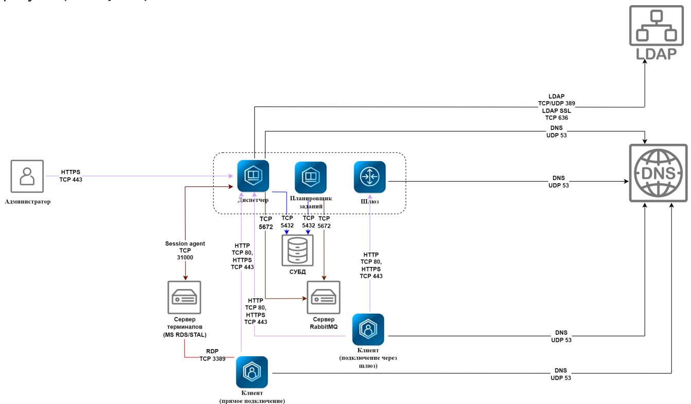
Рисунок 2 – Схема сетевого взаимодействия компонентов Termidesk
