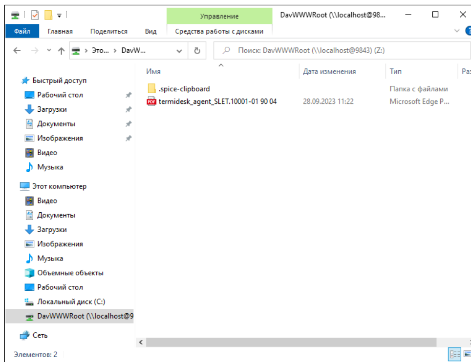
Рисунок 22 – Перенаправленный каталог в ОС Windows
