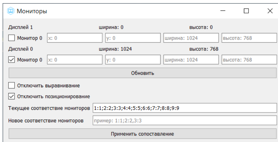
Рисунок 20 – Окно выбора монитора
