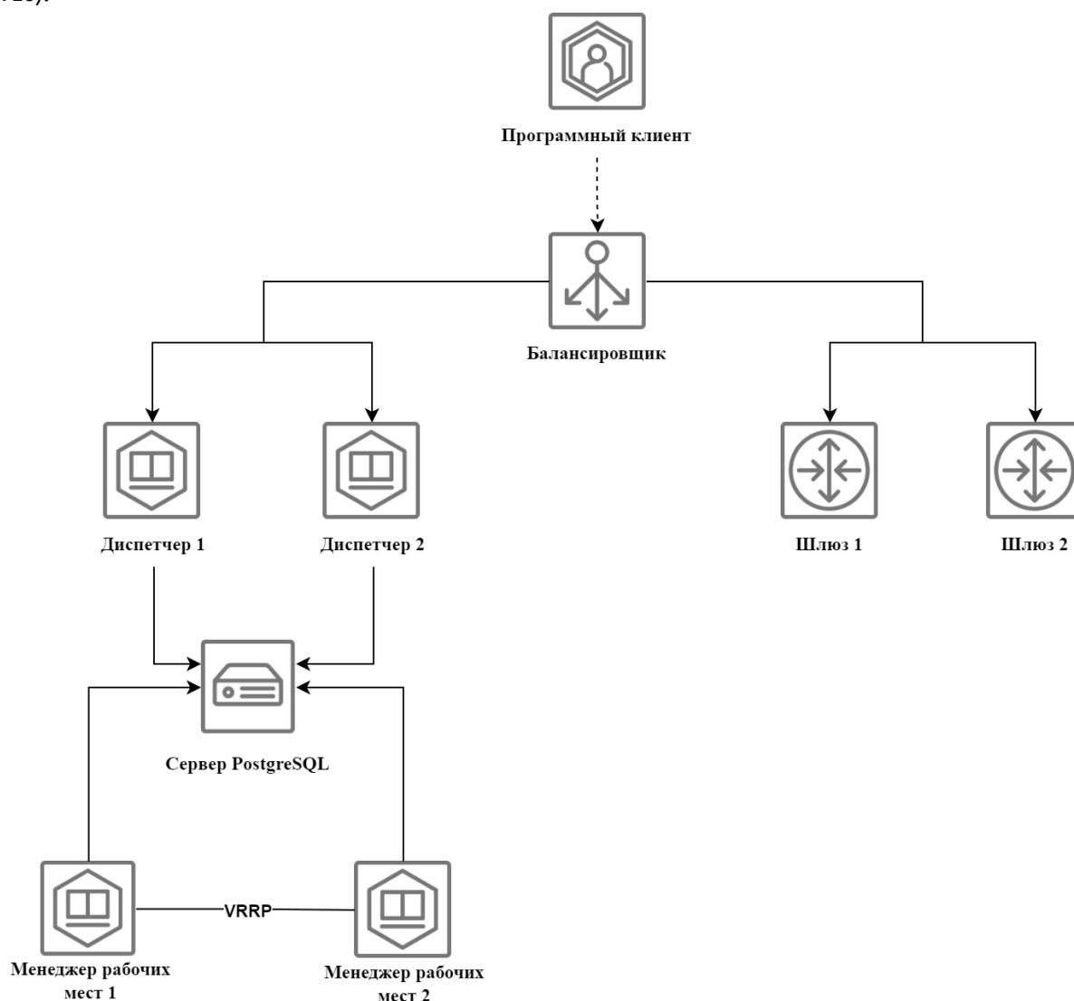
Рисунок 16 – Схема распределенной установки
