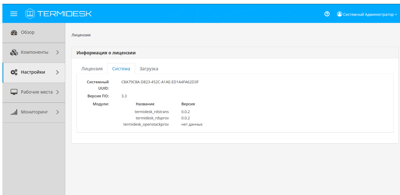
Рис. 4.74 – Информация об уникальном идентификаторе и версии ПО «Диспетчер»
