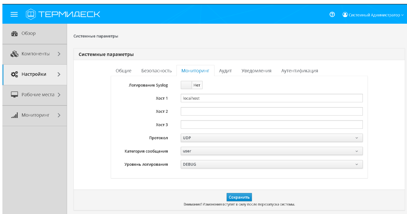
Рис. 4.69 – Настройка системных параметров мониторинга
