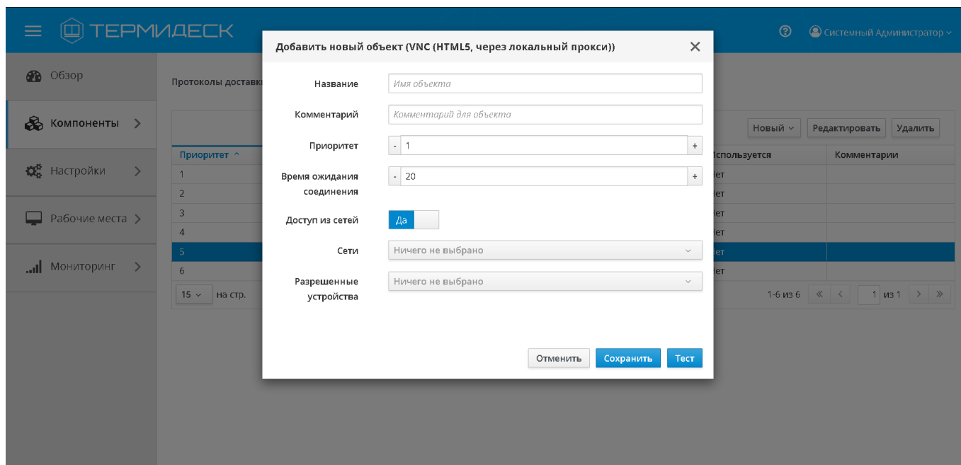
Рис. 4.43 – Добавление подключения по протоколу SPICE через HTML5
