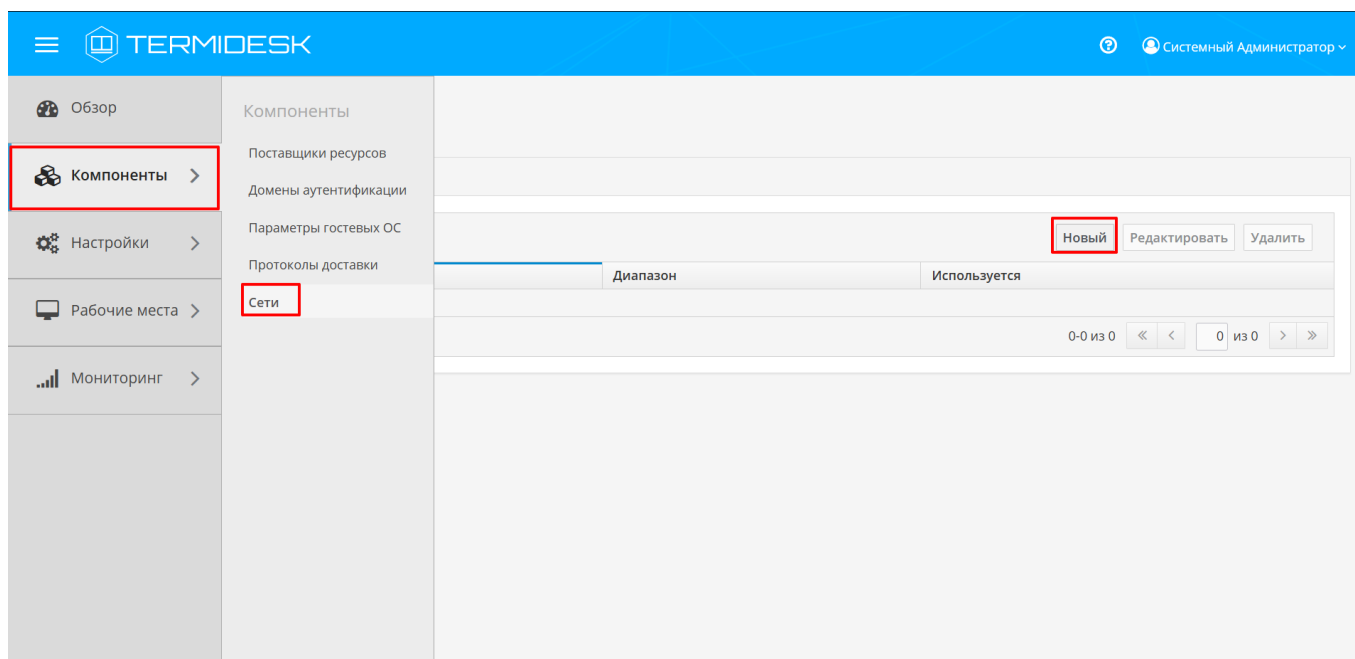
Рис. 4.50 – Добавление аутентификации на основе сетевого адреса
