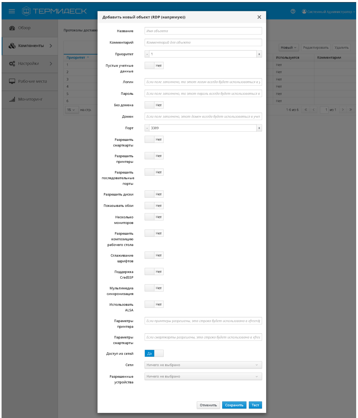
Рис. 4.39 – Добавление прямого подключения по протоколу RDP
