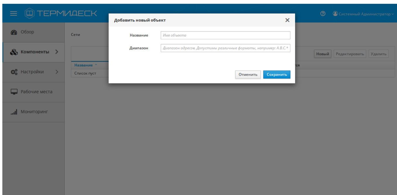
Рис. 4.51 – Добавление адресов сети
