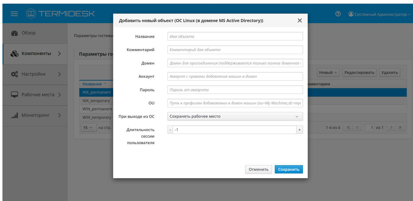
Рис. 4.34 – Добавление параметров гостевой ОС на базе ОС GNU/Linux в домене MS AD (LDAP)
