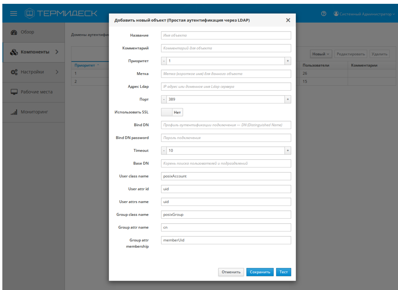
Рис. 4.22 – Добавление параметров LDAP источника сведений
