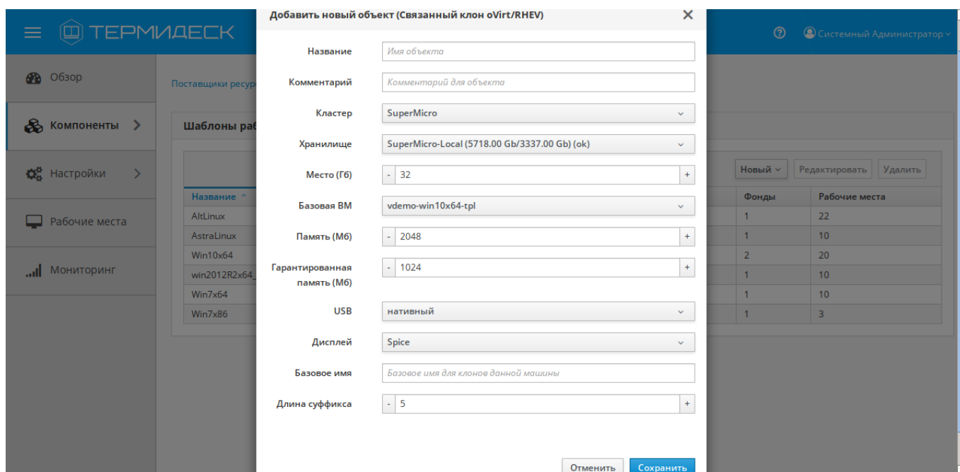
Рис. 4.18 – Добавление связанного клона oVirt/RHEV
