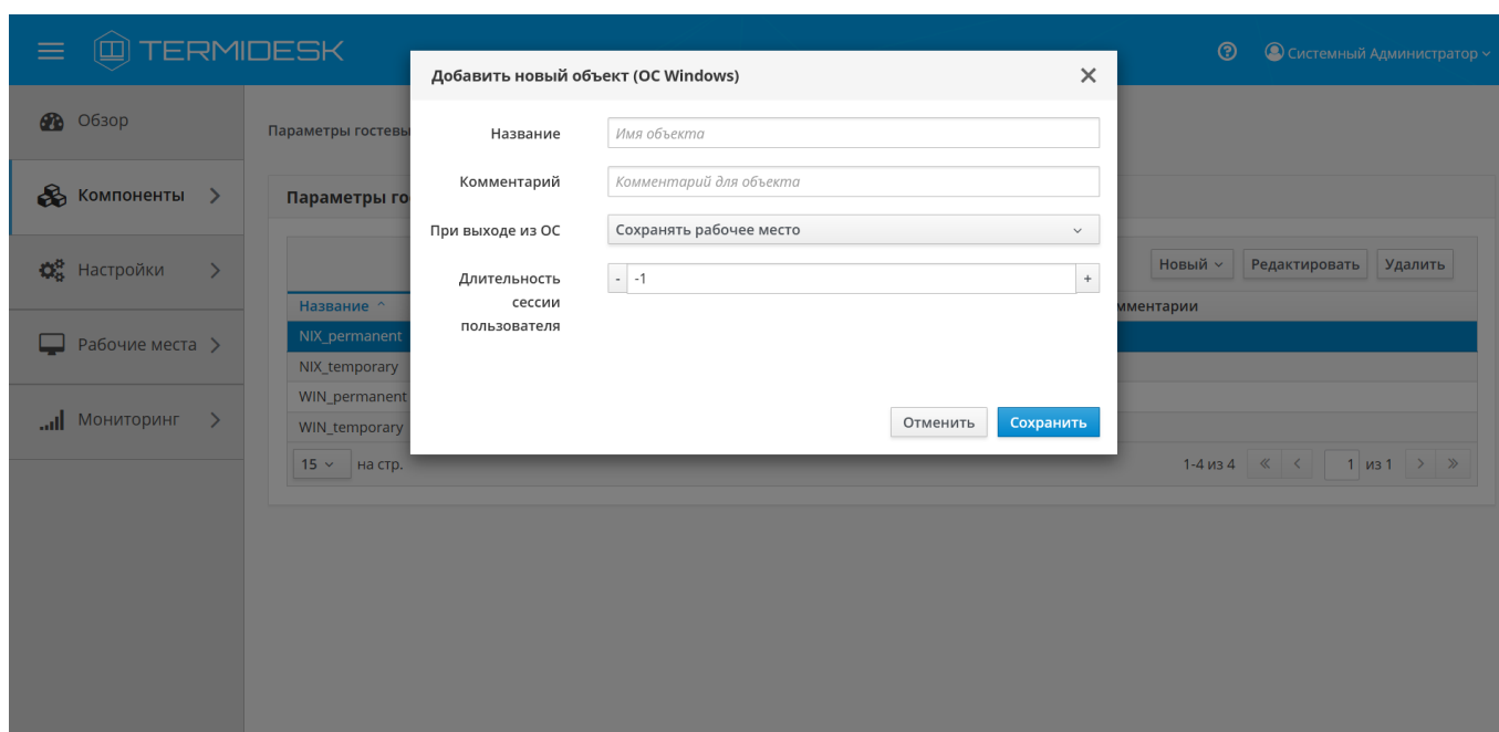
Рис. 4.32 – Добавление параметров гостевой ОС Microsoft Windows без ввода в домен
