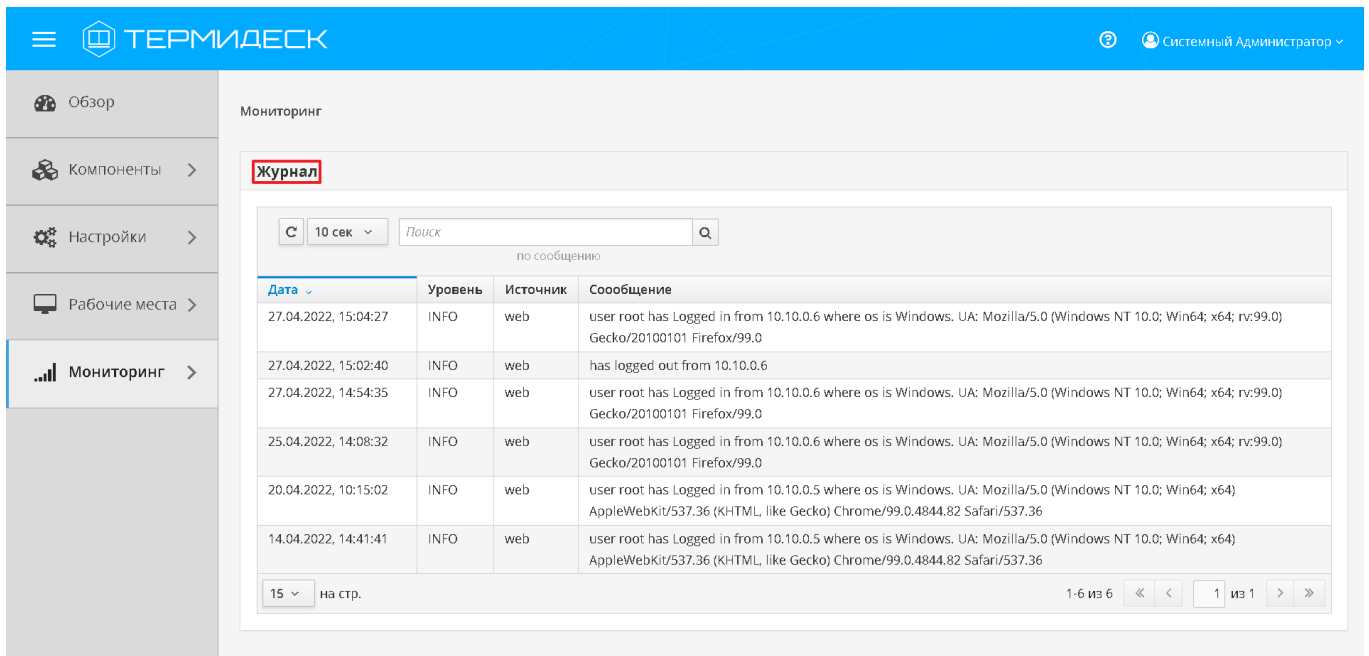
Рис. 4.7 – Процедура «Журнал»
