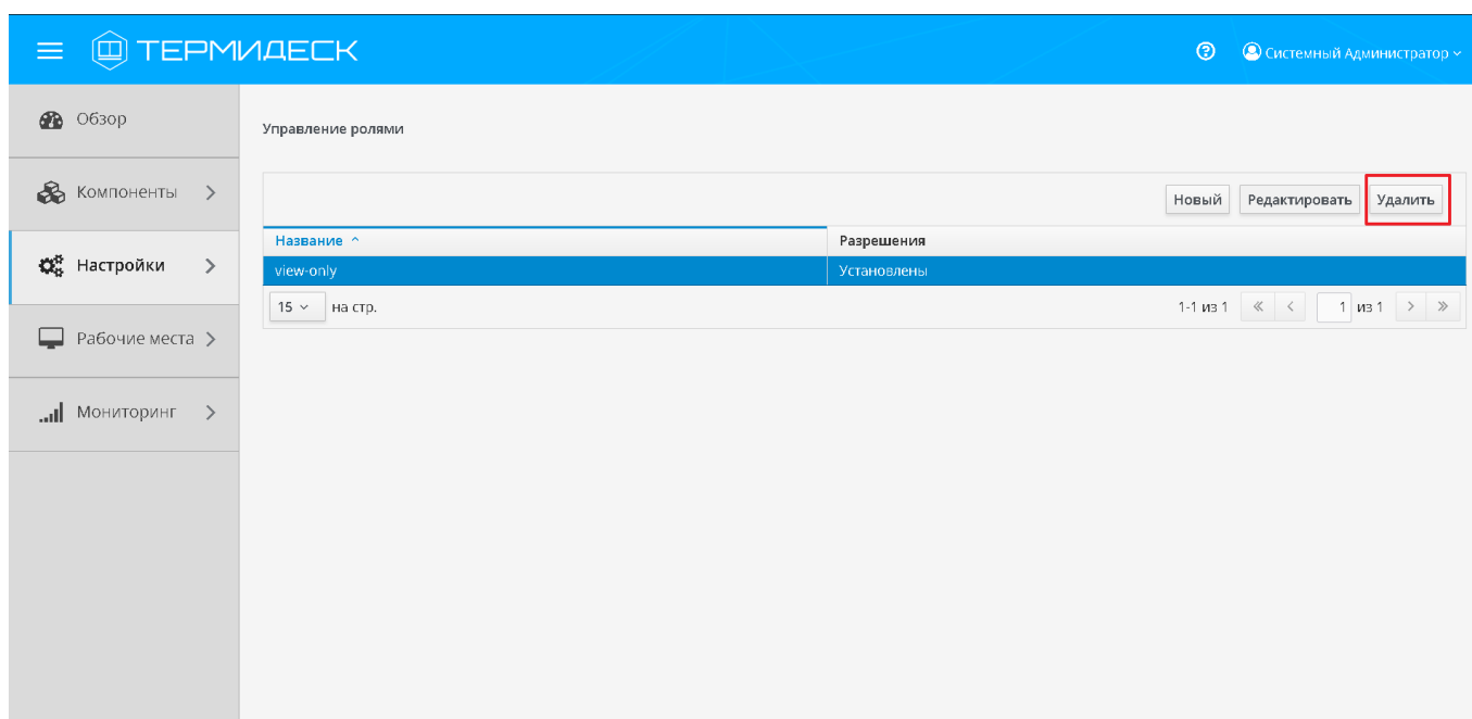
Рис. 4.77 – Удаление роли
