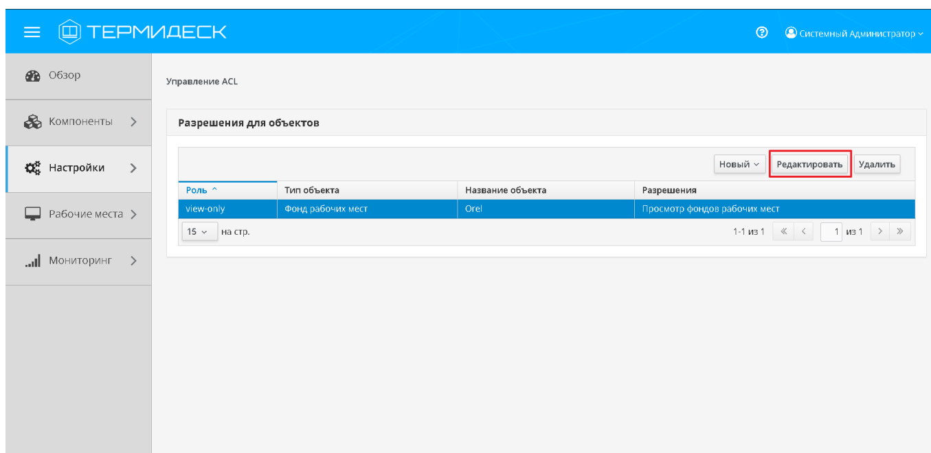
Рис. 4.82 – Редактирование ACL
