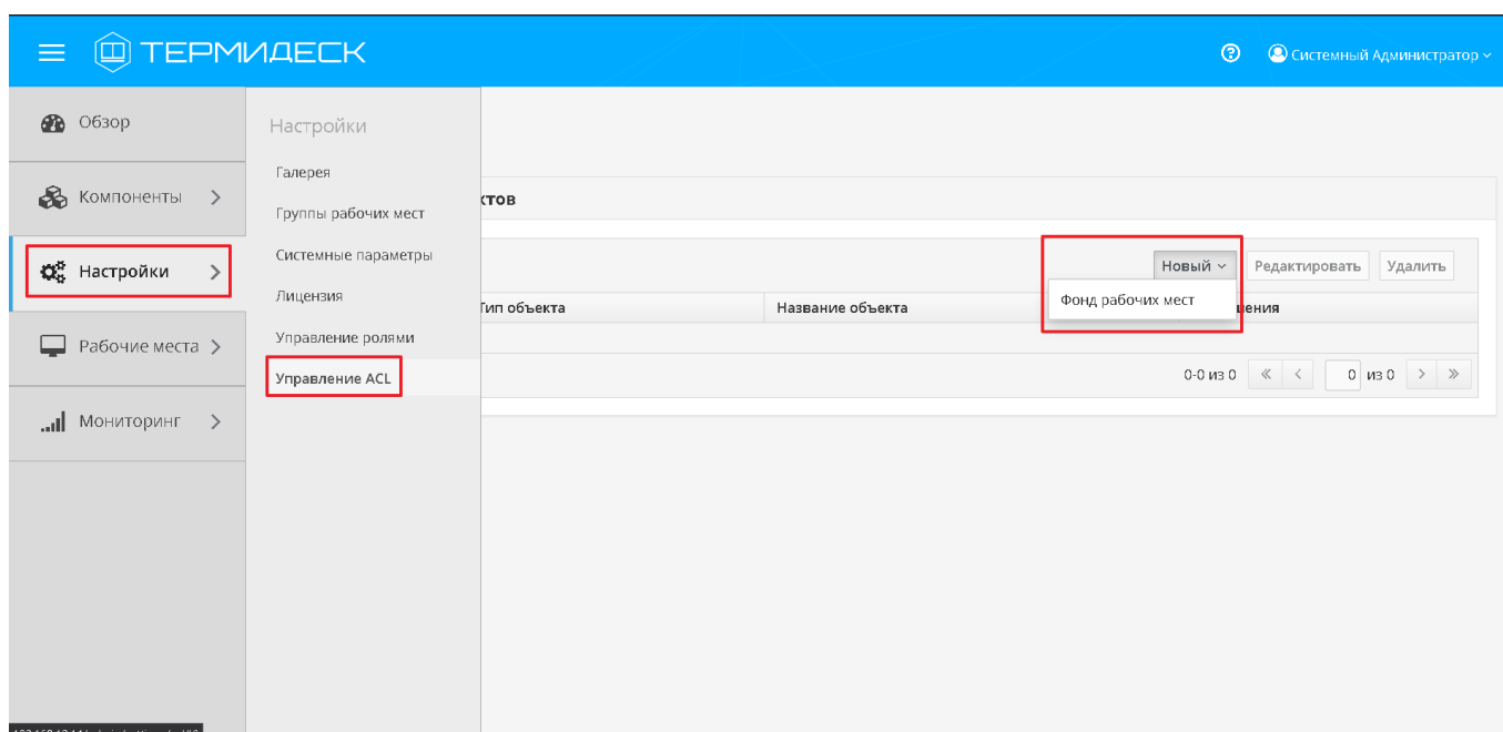
Рис. 4.80 – Добавление ACL
