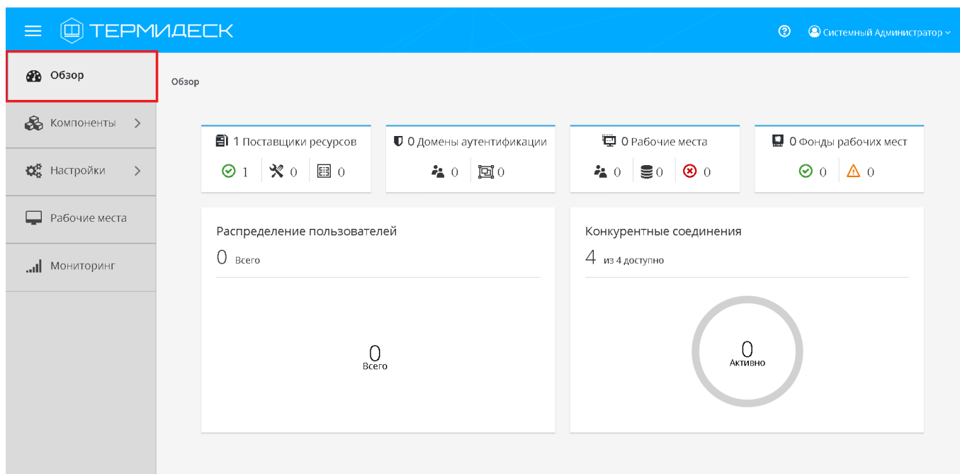
Рис. 4.2 – Функция «Обзор»
