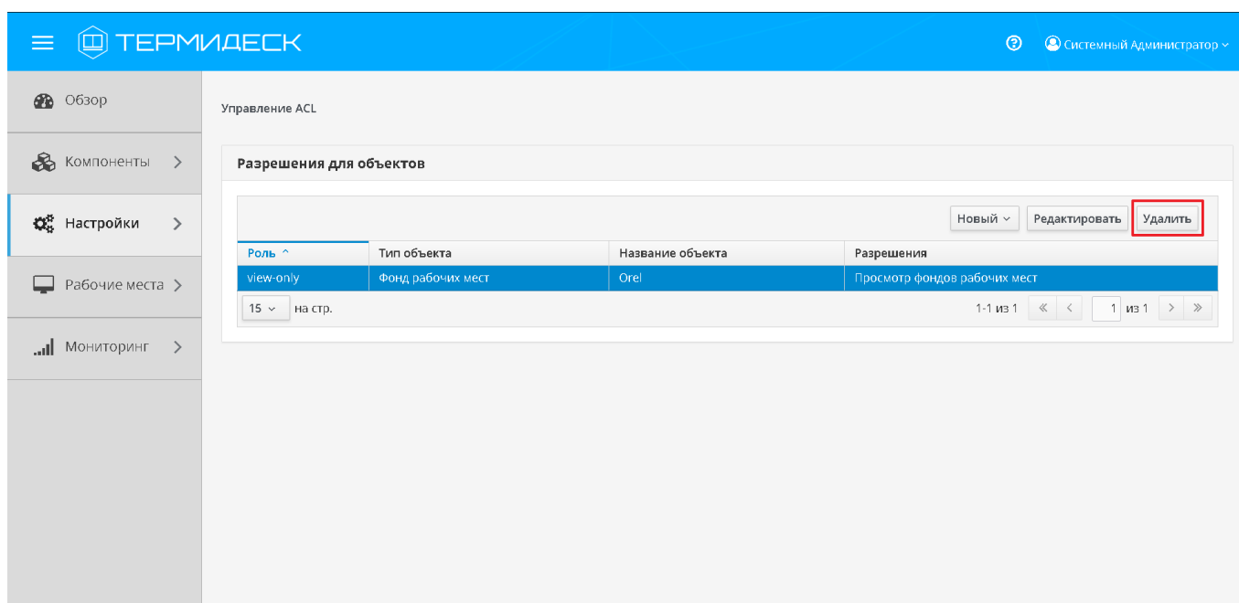
Рис. 4.83 – Удаление ACL
