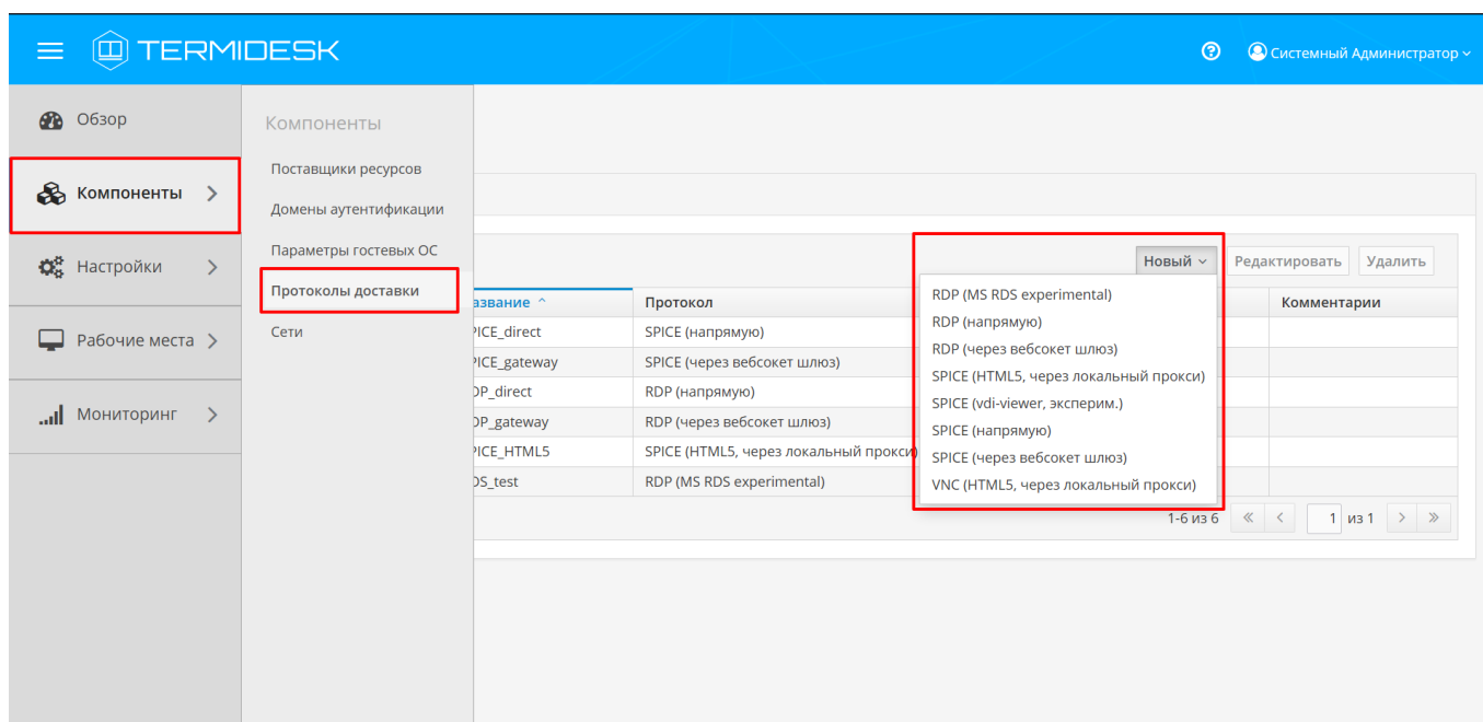
Рис. 4.38 – Добавление протоколов доставки
