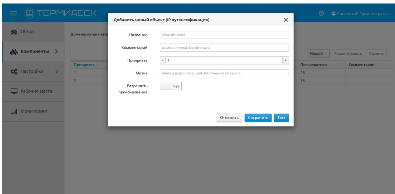
Рис. 4.24 – Добавление аутентификации по IPv4-адресам
