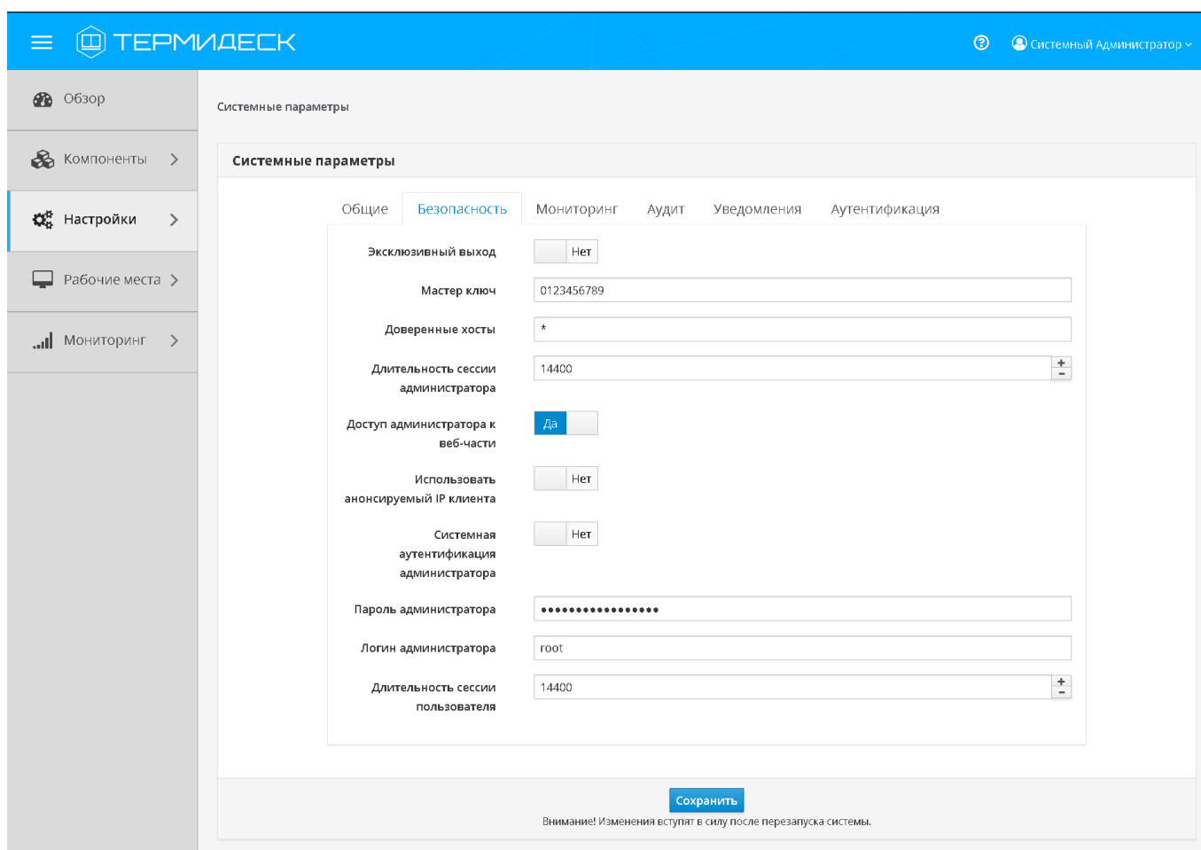
Рис. 4.68 – Настройка системных параметров безопасности
