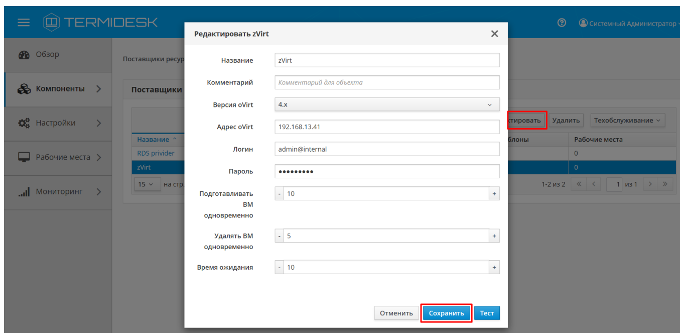
Рис. 4.13 – Редактирование поставщика ресурсов
