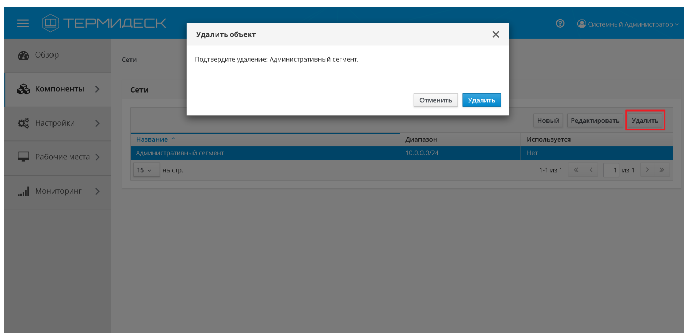
Рис. 4.53 – Удаление аутентификации на основе сетевого адреса
