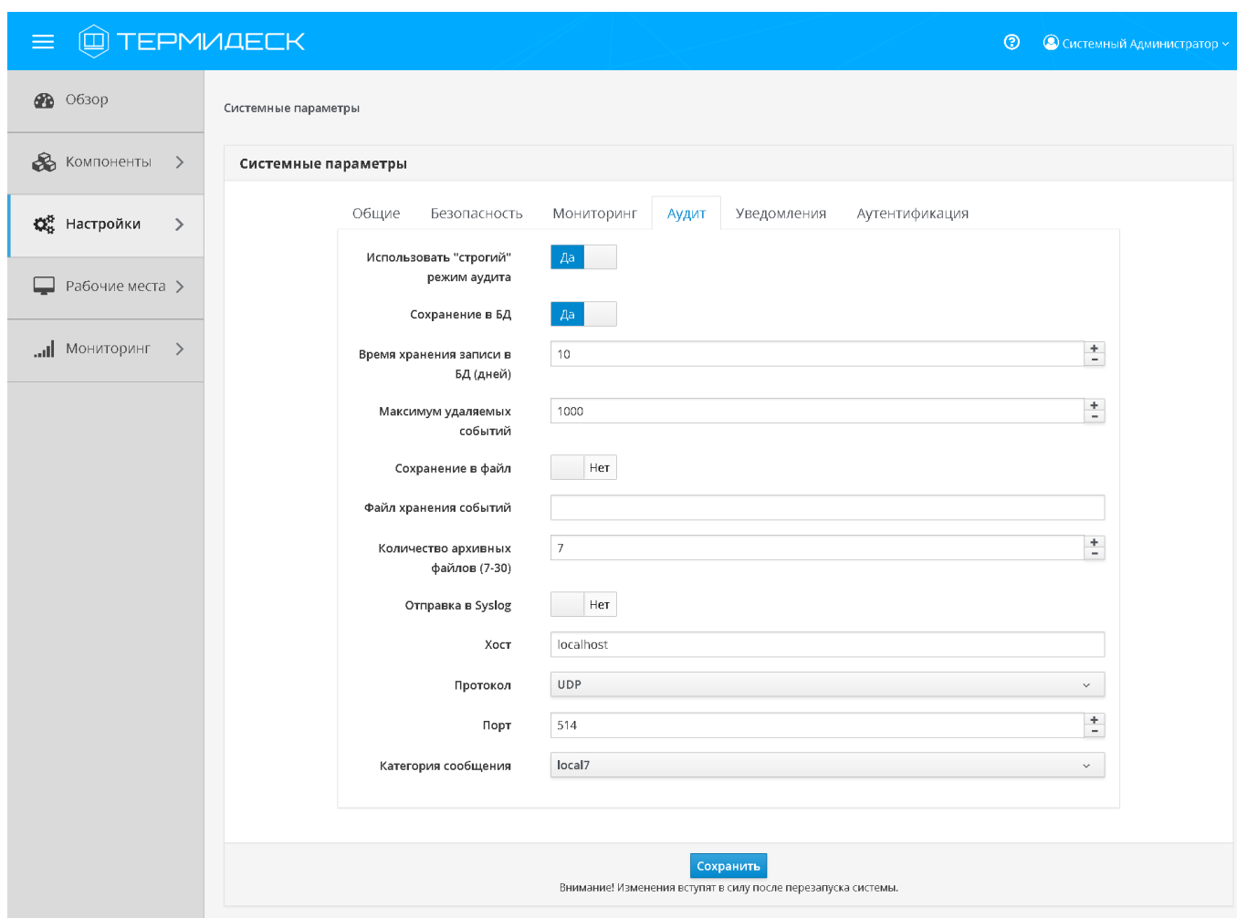
Рис. 4.70 – Настройка регистрации событий системного аудита
