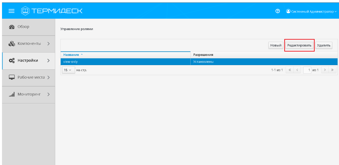
Рис. 4.76 – Редактирование роли
