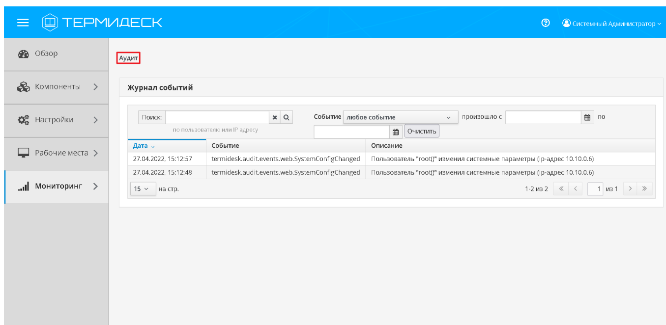
Рис. 4.8 – Процедура «Аудит»
