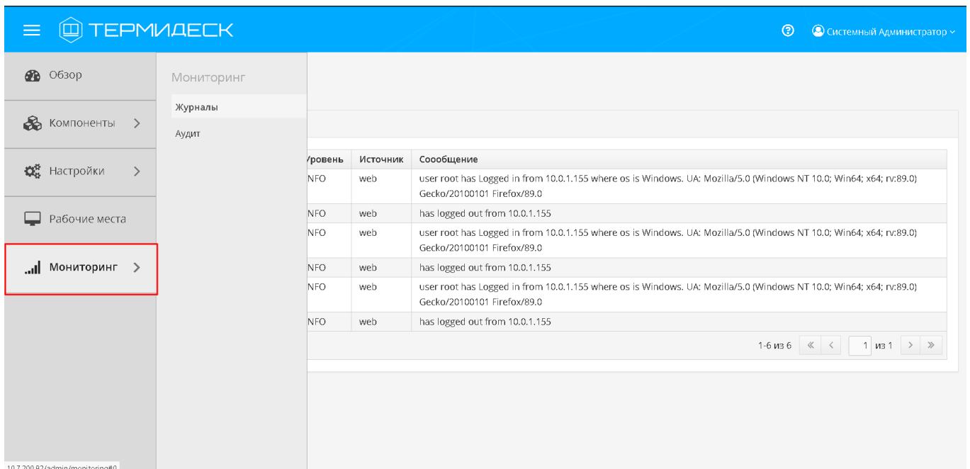
Рис. 4.6 – Функция «Мониторинг»
