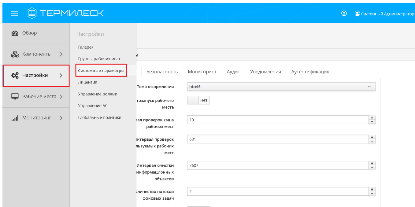
Рис. 4.65 – Системные параметры
