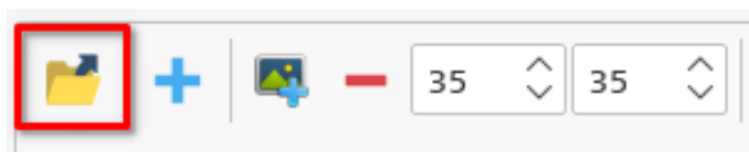
Рис. 31
